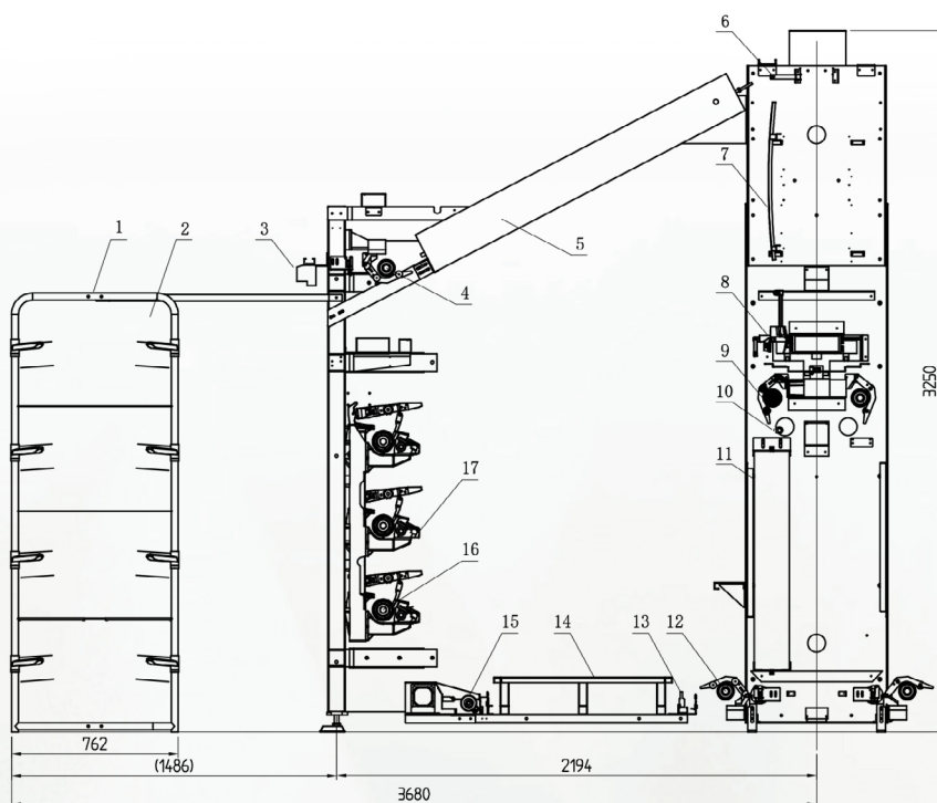
【外形尺寸示意图】 Overall dimension
