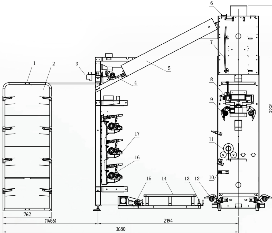
【外形尺寸示意图】 Overall dimension
